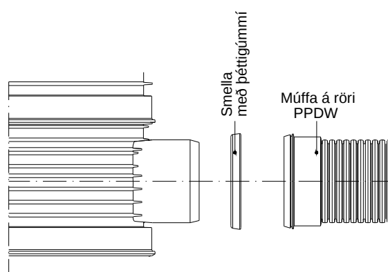
Samsetning við brunnstúta 200mm og minni
