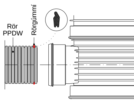
Samsetning við brunnstúta 250mm og stærri
